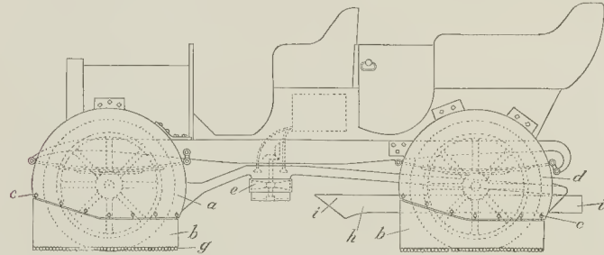
Aparato para suprimir las molestias del polvo, de las salpicaduras de barro y del humo de los automóviles, motocicletas y tranvías, inventado por el Sr. Josephanes, de Barcelona
